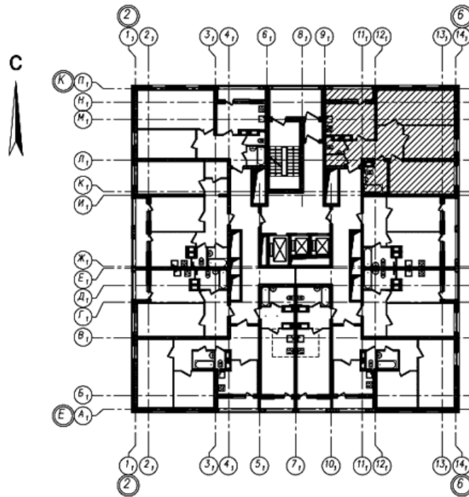
Проектные характеристики Объекта строительства (многоквартирного дома)
